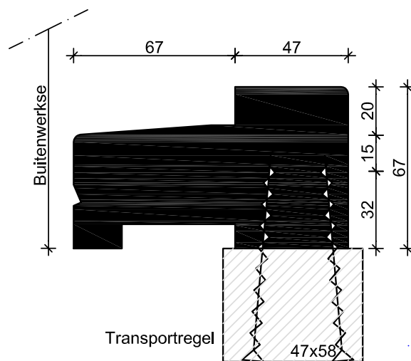
Onderdorpel
