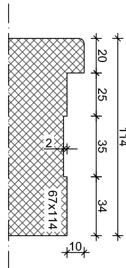
Kantstijl
