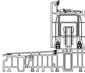
binnenzijde schuivend
