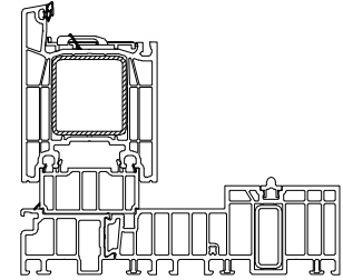
buitenzijde vast
