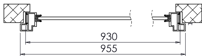
SECTION B-B SCALE 1 : 5
