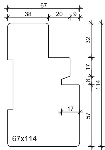
Draaikiepsponning - Draaikiepraam
