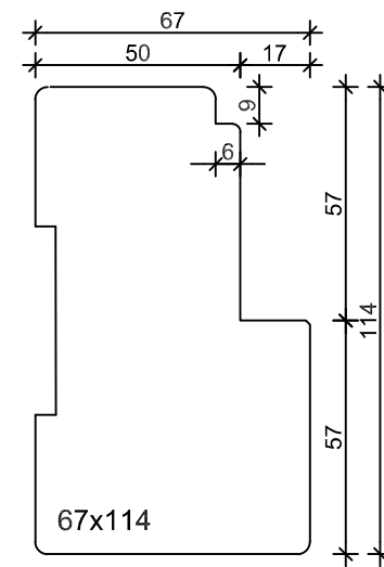
Binnensponning + voorsponning - Binnendraaiende deur
