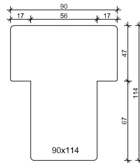
Buitensponning - Buitendraaiende deur - Draairaam - Uitzetraam
