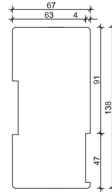
Schuifpui sponning - Schuifpui
