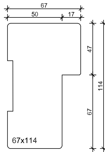
Buitensponning - Buitendraaiende deur - Draairaam - Uitzetraam
