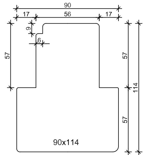
Wisselspanning Binnendraaiende deur - vast glas / paneel
