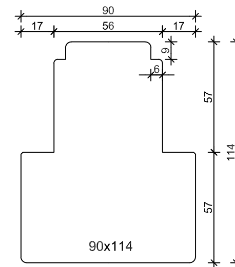
Binnensponning + voorsponning - Binnendraaiende deur
