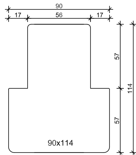
Binnensponning - Vast glas - Paneelvulling
