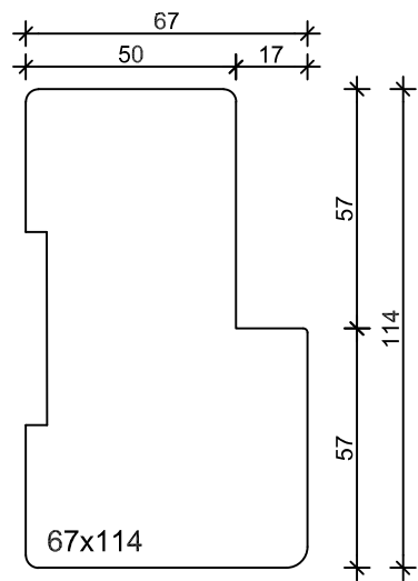
Binnensponning - Vast glas - Paneelvulling
