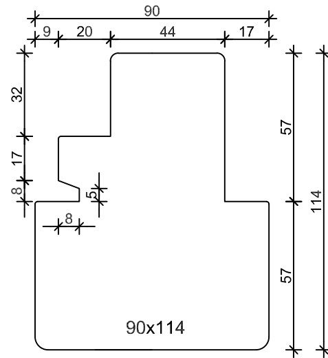
Wisselspanning Draaikiepraam - vast glas / paneel
